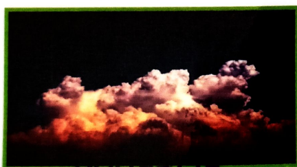
КУЧЕВЫЕ
