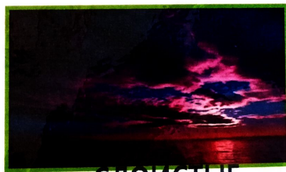
СЛОИСТЫЕ
